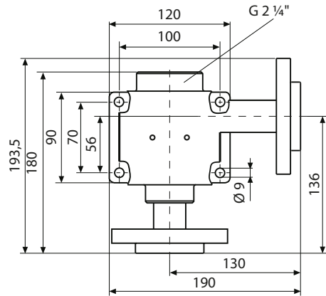
DN 25 flange, 90°
